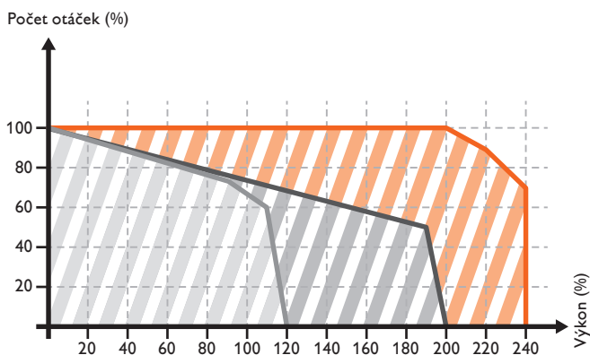
Srovnání charakteristik otáček podle výkonu:
