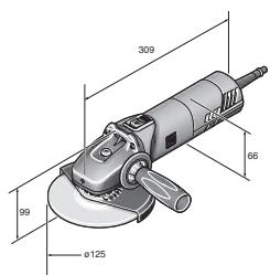
WSG 17-70 Inox Základní sada WSG 17-70 Inox
